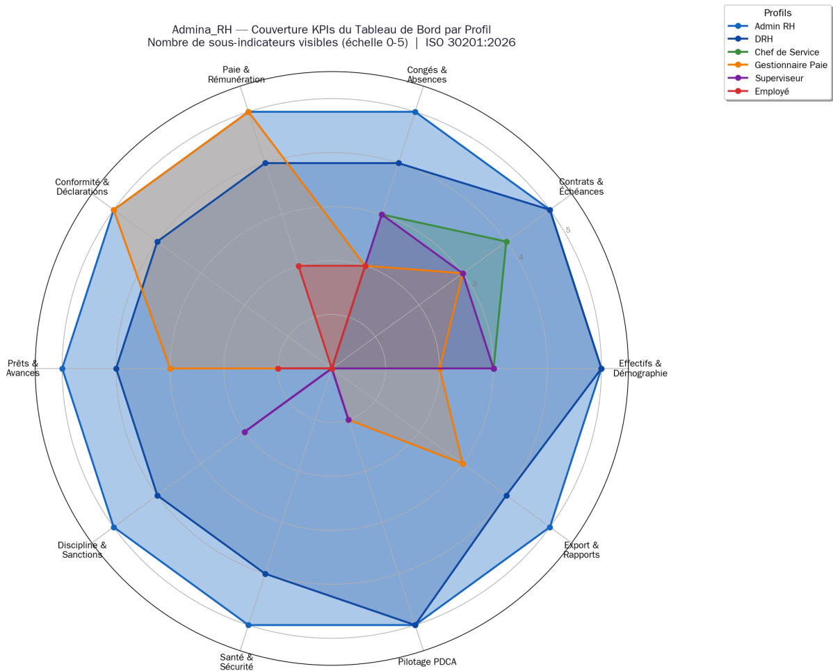
Figure 4-1 : Couverture des KPIs du Tableau de Bord par profil utilisateur
